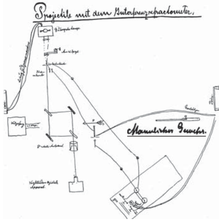
Spätere Versuchsanordnung Ernst Machs (um 1893 - man beachte „Mannlichergewehr“)
