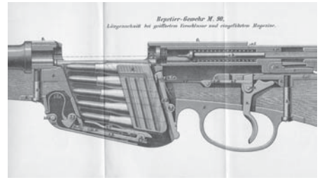
Systemschnitt des österreichischen Repetiergewehrs M.1890 System Mannlicher, Kal. 8mm
